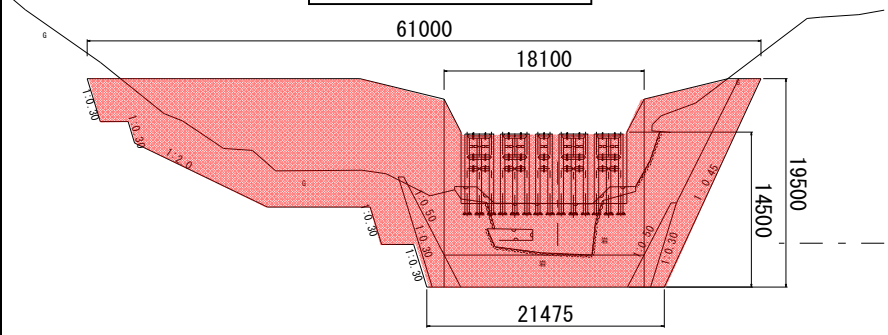
2号堰堤正面図
