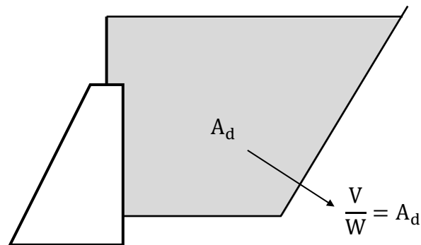
図 2-38 単位幅当たりの崩壊土量 A_d (m 2 ) の算出
