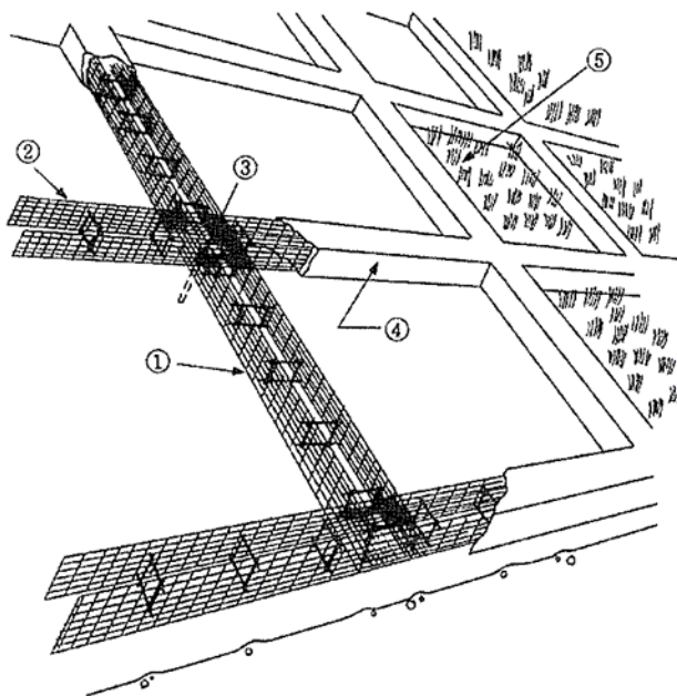
図 2-19 吹付砕工施工の一例
