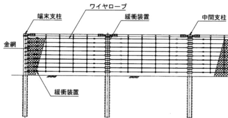
図 2-41 待受式高エネルギー吸収型崩壊土砂防護柵工
