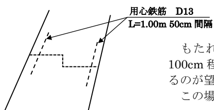
図 2-32 断面図（参考）
