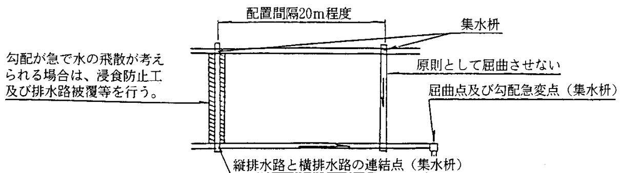
図 2-8 縦排水路の配置(平面図)
