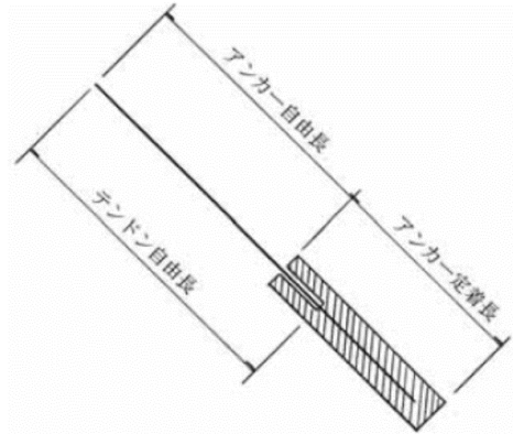
図 2-51 アンカーの各長さ
