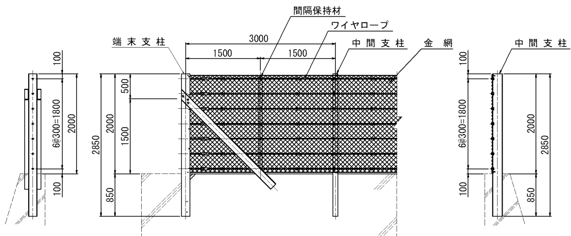
図 2-60 落石防護柵の構造例
