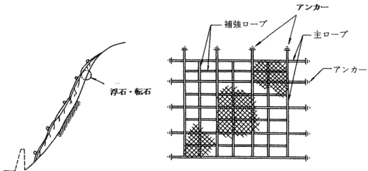
図 2-57 覆式落石防護網の例
