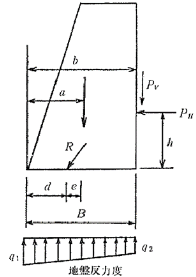
図 2-33 地盤反力度の求め方
