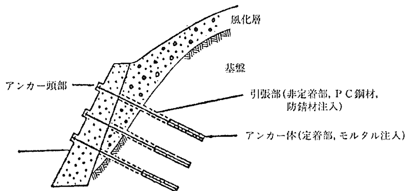
図 2-43 斜面アンカー工の例（擁壁の捕強）
