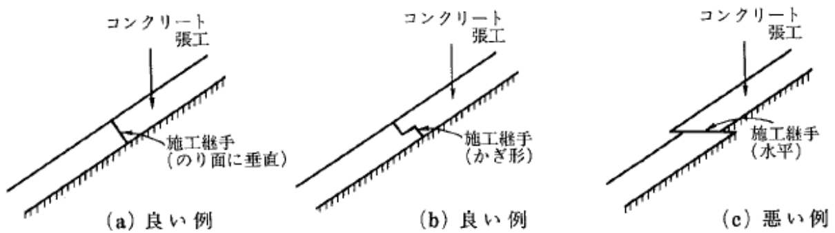
図 2-16 コンクリート張工の例
