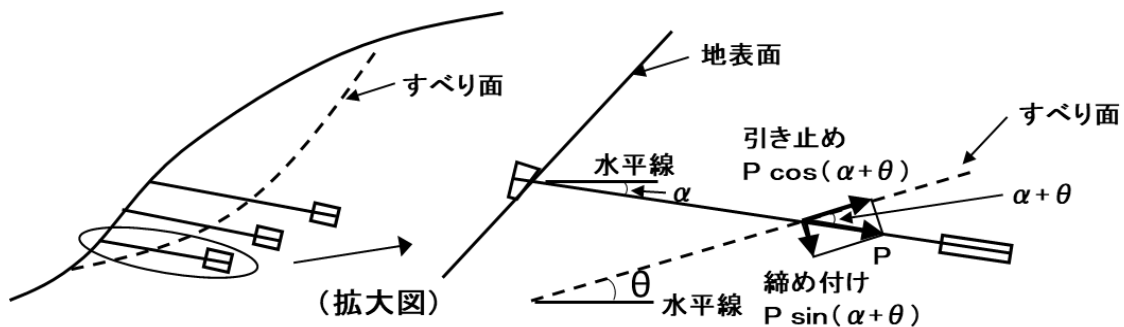
図 2-47 引き止め機能を期待する場合（すべり面の勾配が緩い場合）
