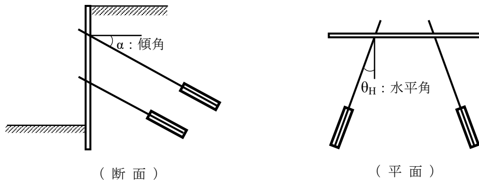
図 2-49 アンカー傾角・水平角
