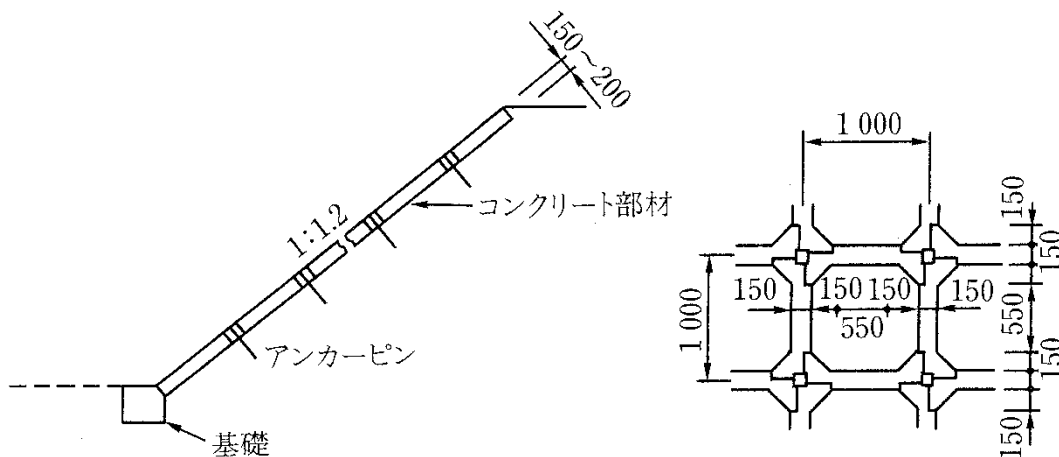
図 2-21 プレキャストのり枠工の例（単位：mm）
