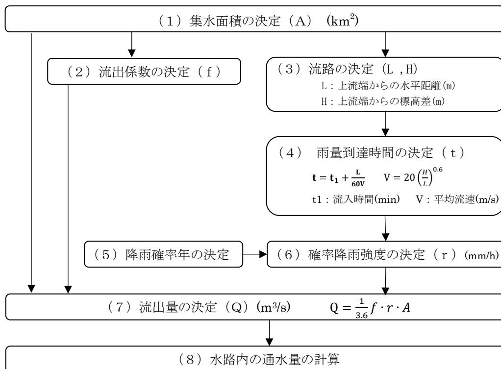
図 2-2 雨量流出量の算定手順
