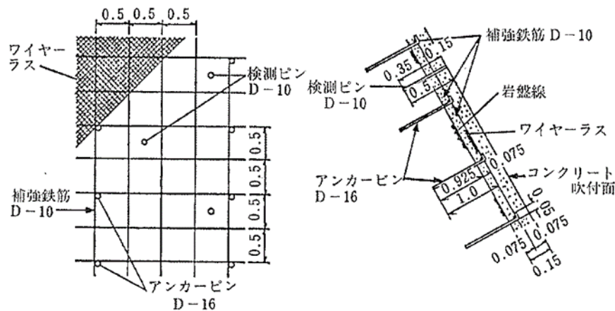
図 2-14 コンクリート吹付工の一例(単位：m)
