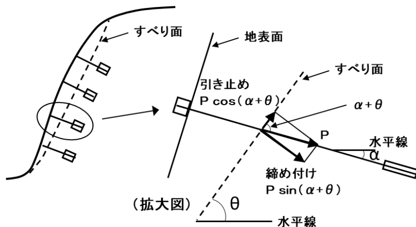
図 2-46 締め付け機能を期待する場合（すべり面の勾配が急な場合）
