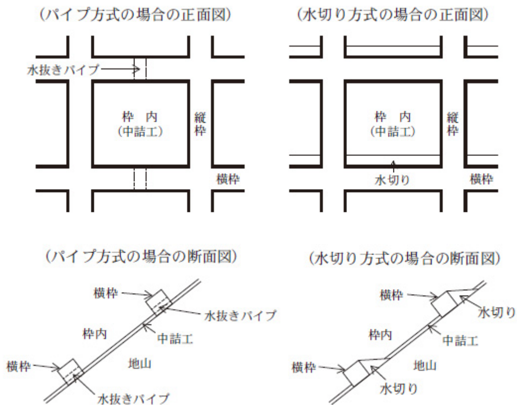
図 2-23 現場吹付のり枠工の枠内排水方法に関する概念図
