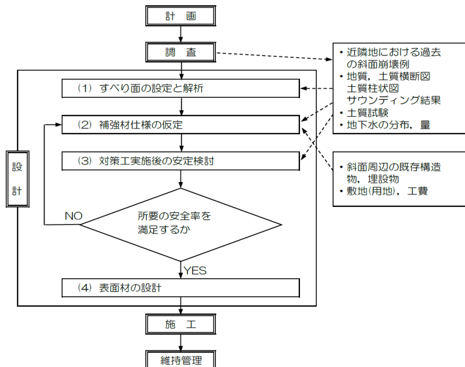
図 2-53 地山補強土工の一般的な設計手順
