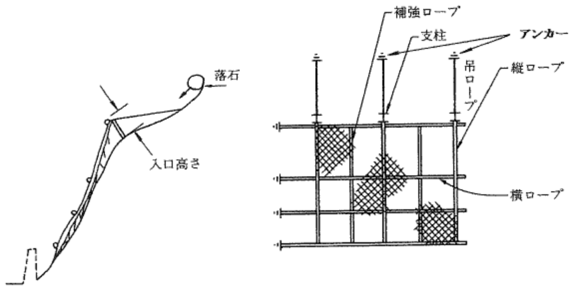
図 2-58 ポケット式落石防護網の例
