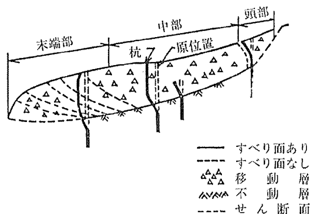
図 2-62 地すべりと杭の概念図
