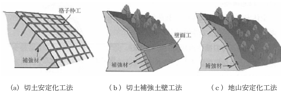
図 2-52 地山補強土工の種類
