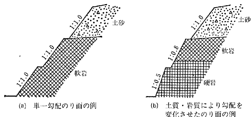
図 2-24 地山状態とのり面形状の説明図
