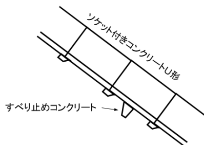
図 2-5 縦排水路（すべり止めコンクリート付）
