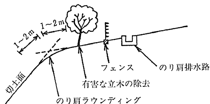
図 2-25 のり肩部処理
