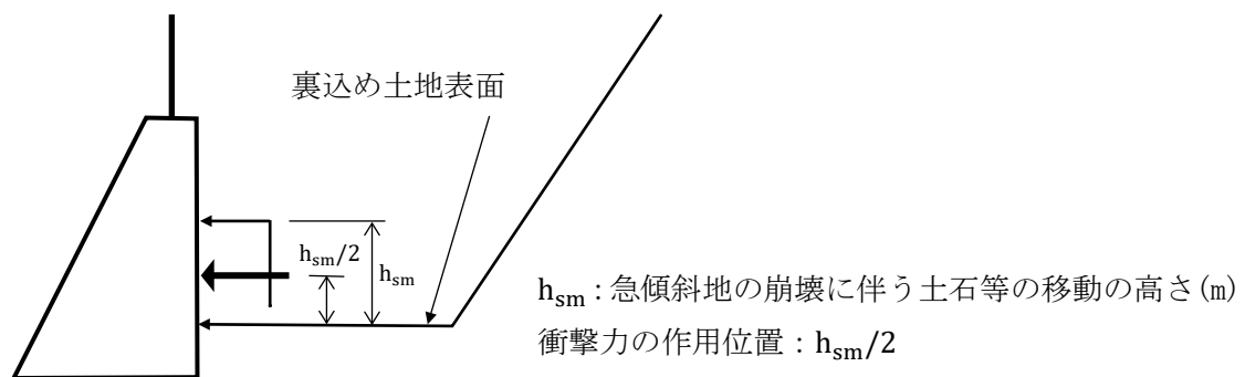
図 2-36 衝撃力作用位置
