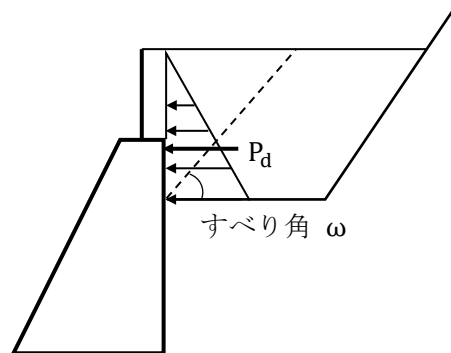
(a) 崩壊土砂による土圧
