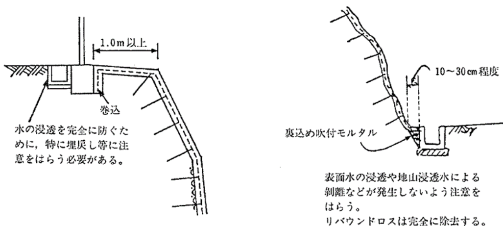
図 2-15 のり肩の処理の一例（左）とのり尻の処理の一例（右）
