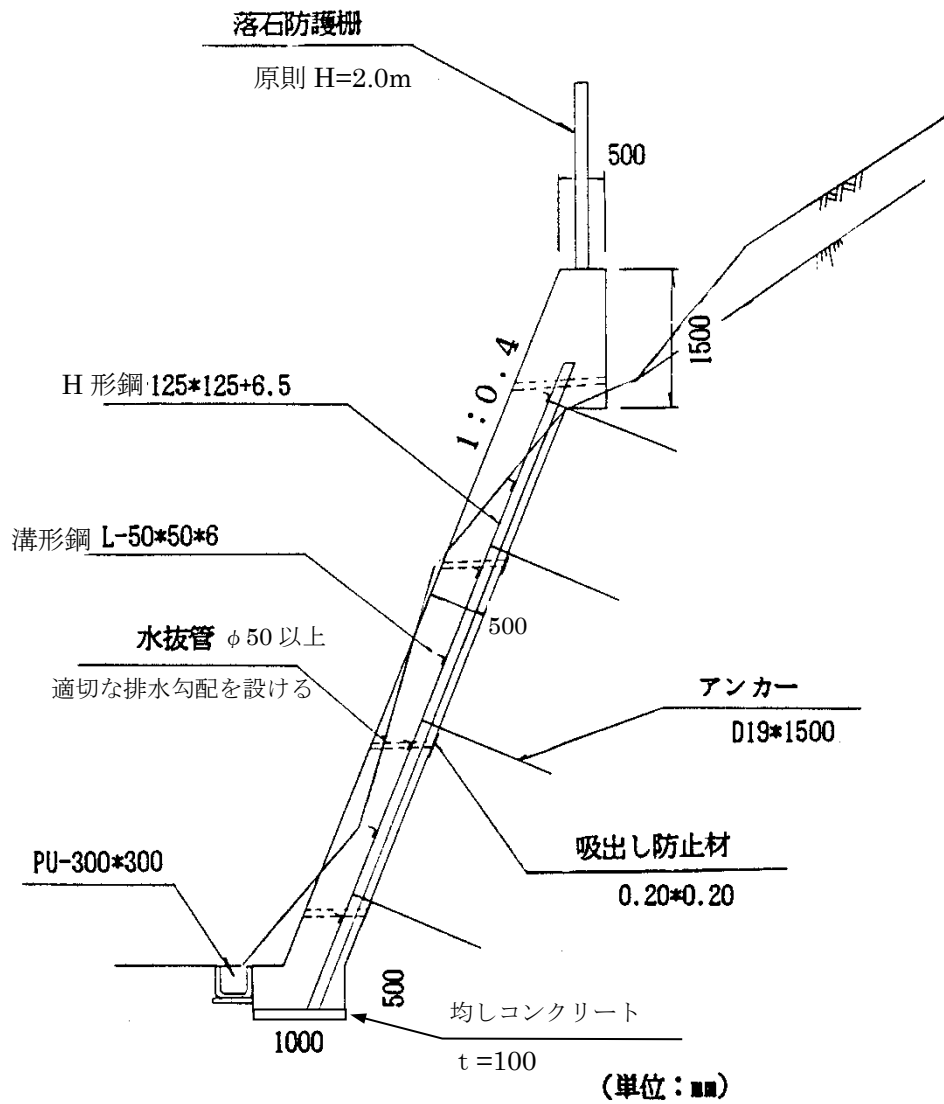
図 2-16 コンクリート張工の例
