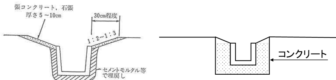
図 2-6 縦排水路の跳水対策
