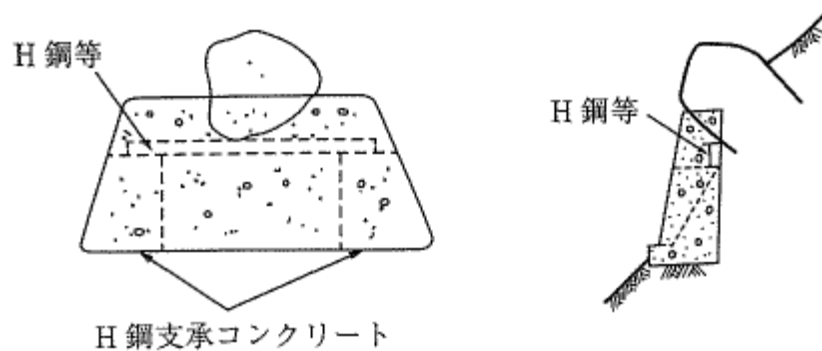
図 2-55 コンクリート根固工の例
