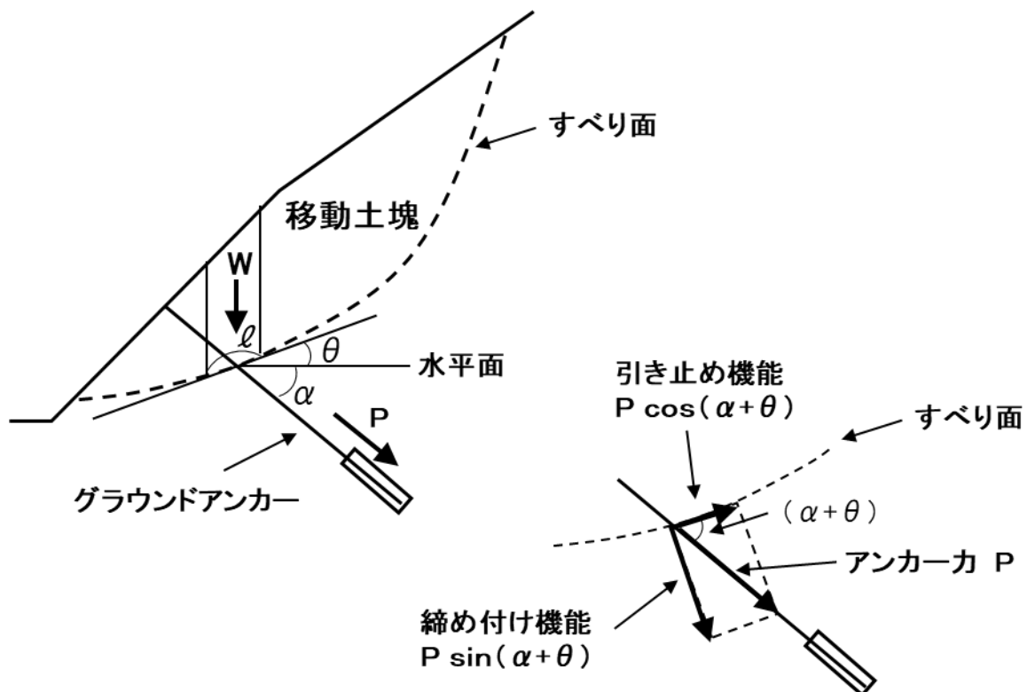
図 2-50 アンカーの抑止機能
