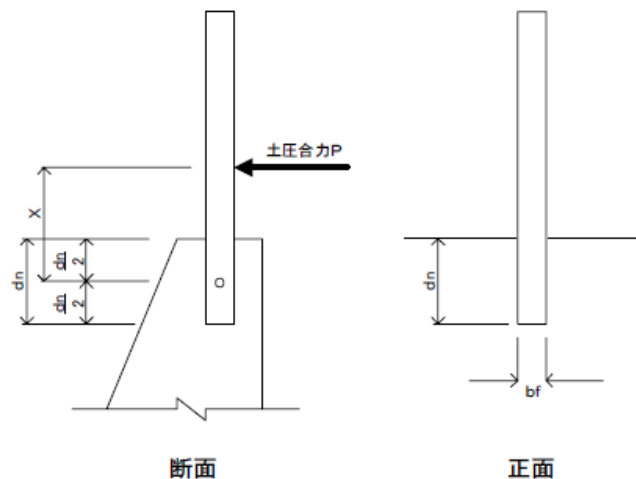
図 5-1 支柱根入れ部
