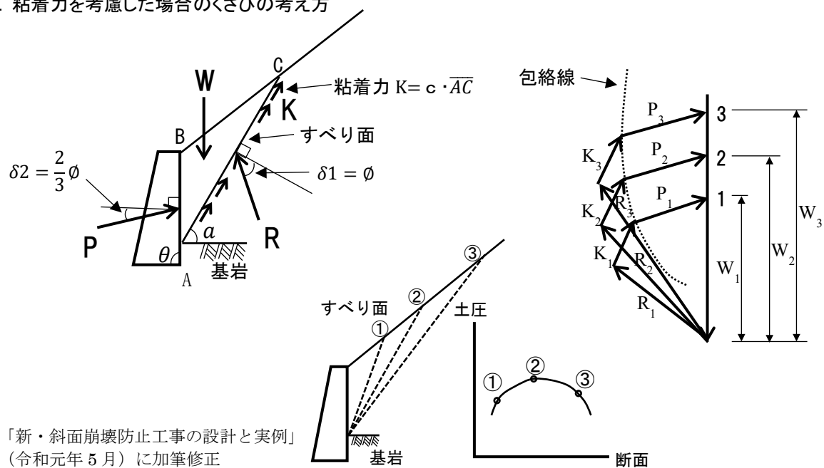
図 2-31 直試行くさび法による土圧の算定
