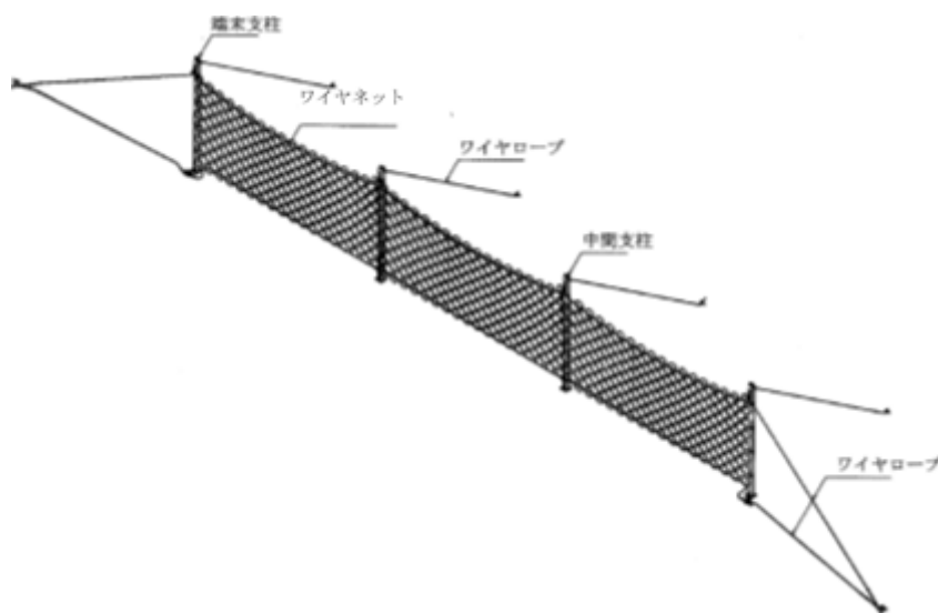
図 2-42 柔構造斜面崩壊対策待受け工
