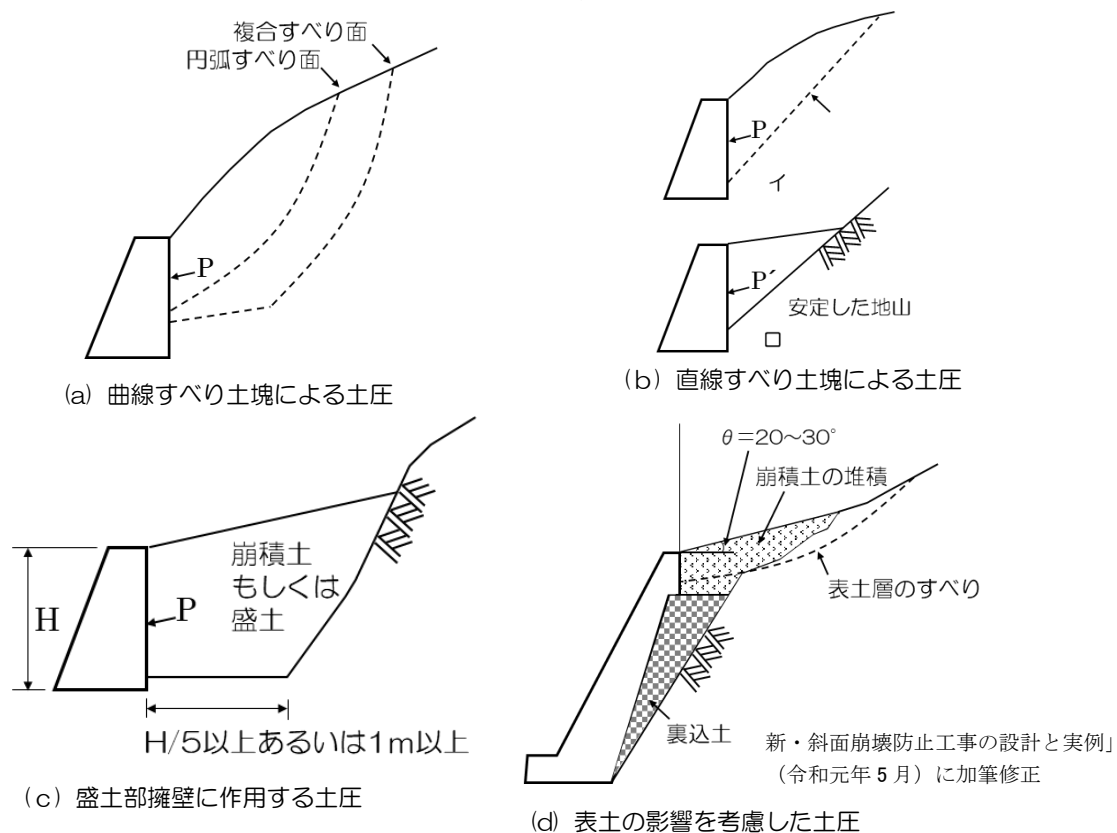
図 2-27 斜面における土圧の分類
