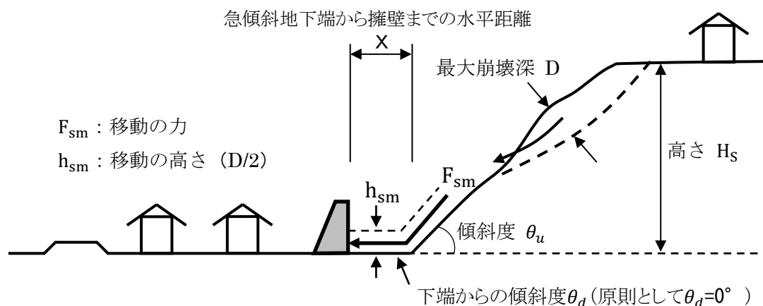
図 2-35 土砂崩壊と移動の力のイメージ
