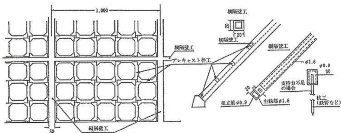
図 2-21 プレキャストのり枠工の例（単位：mm）
