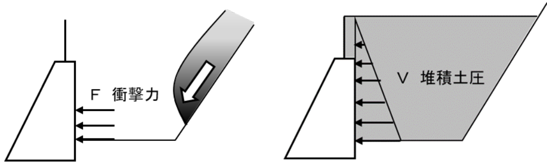
図 2-40 擁壁に作用する力
