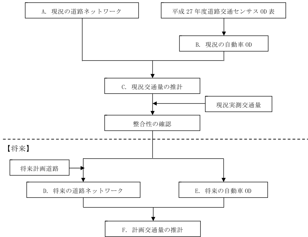
図 3.3-2 計画交通量推計手順
