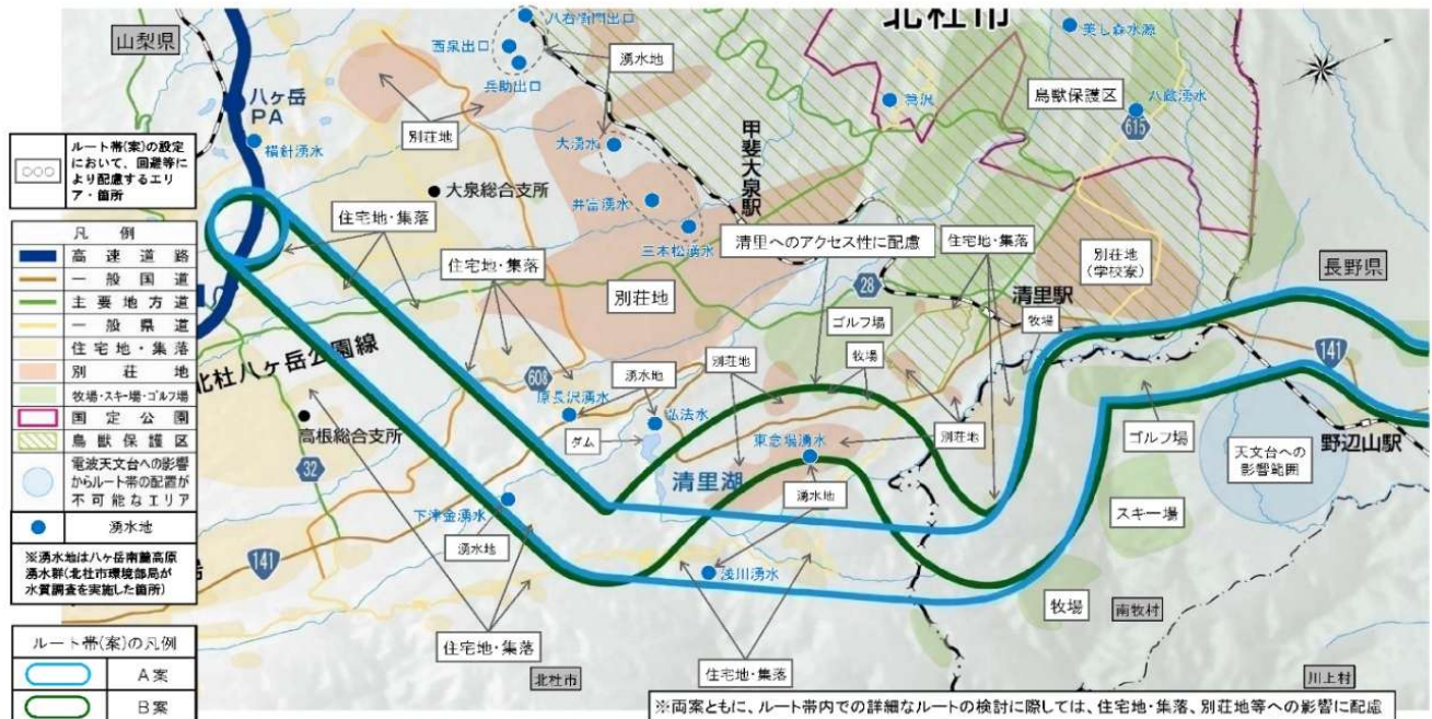
図 3.4-3 設定したルート帯案の概要
