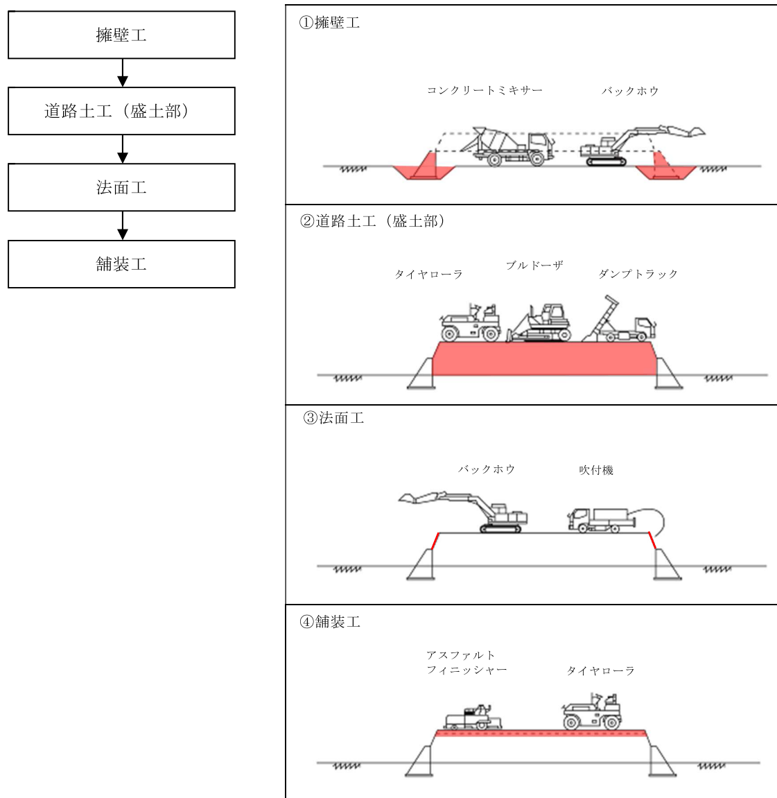
図 3.3-6 土工工事（盛土部）の施工順序
