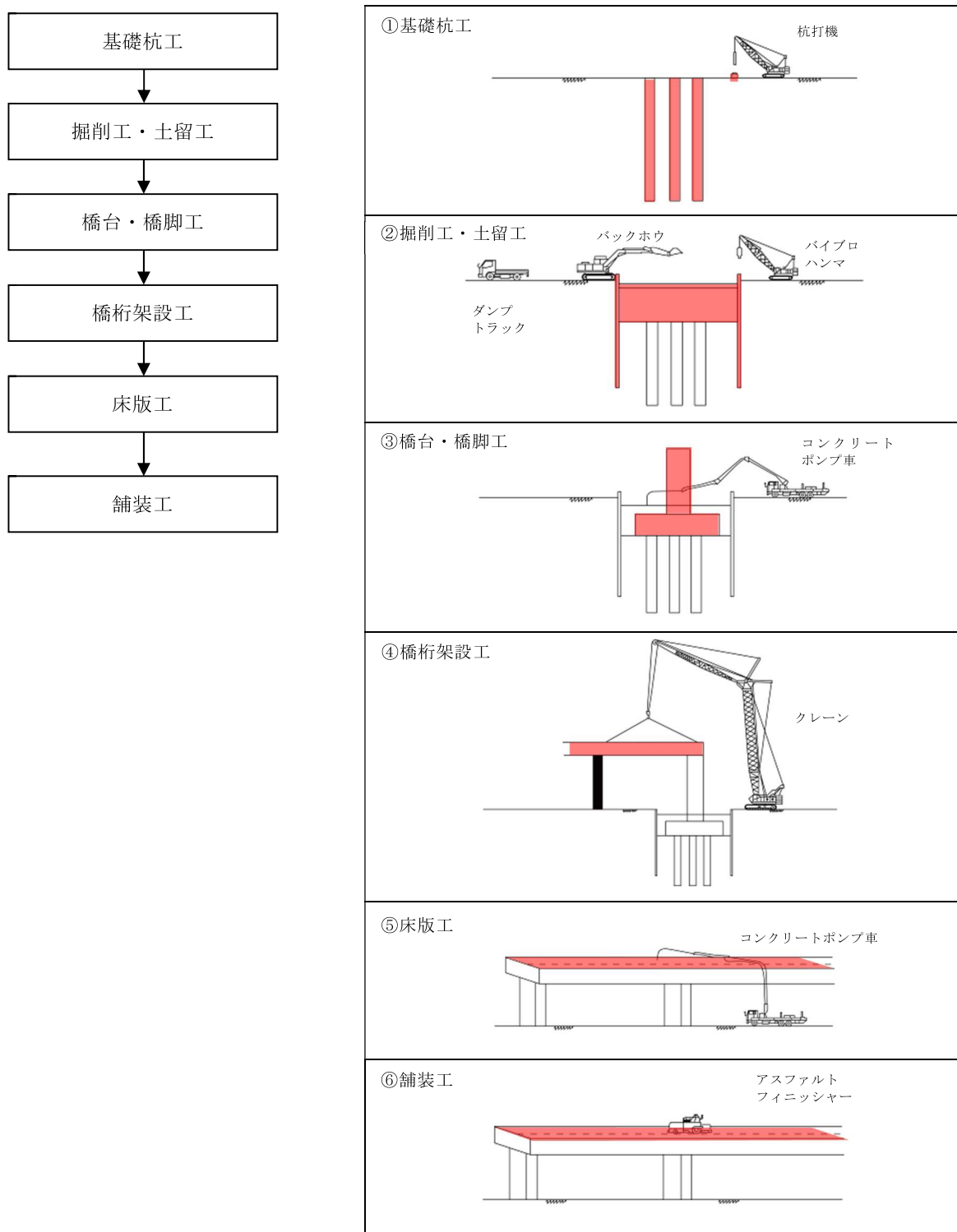
図 3.3-8 橋梁工事の施工順序
