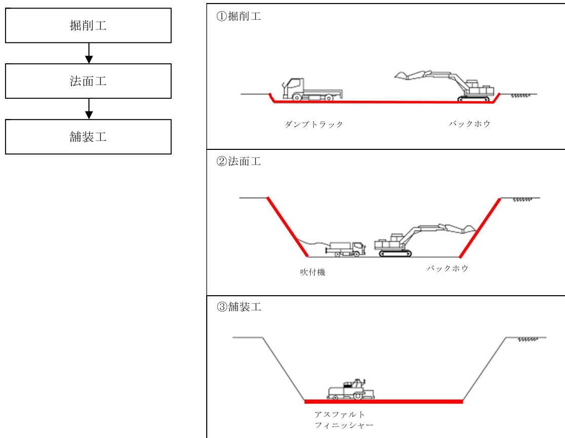
図 3.3-7 土工工事（切土部）の施工順序
