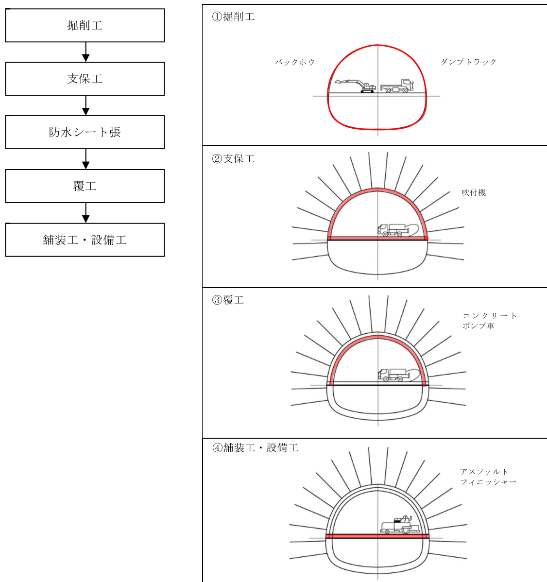
図 3.3-9 トンネル工事の施工順序
