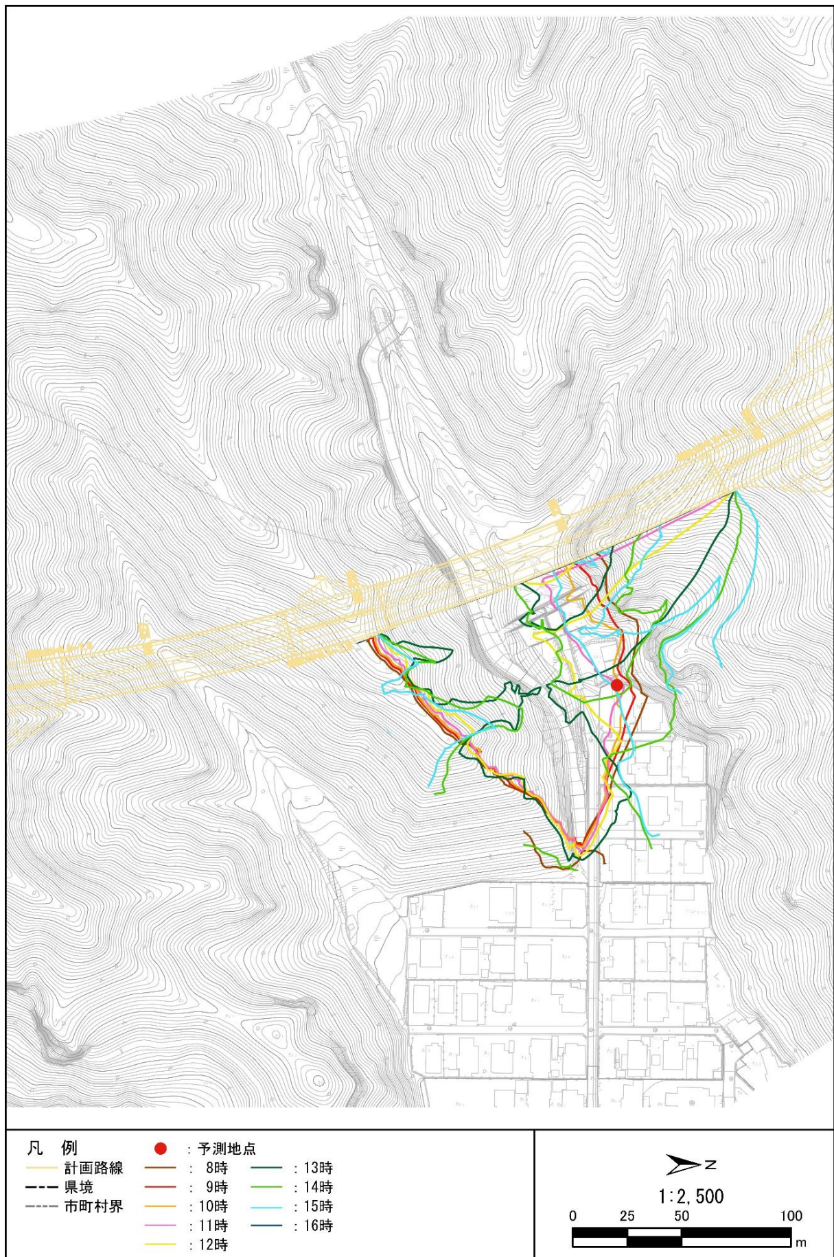
図 6.1-2 (6) 等時刻日影図 (N6. 小海町豊里 4) (長野県)
