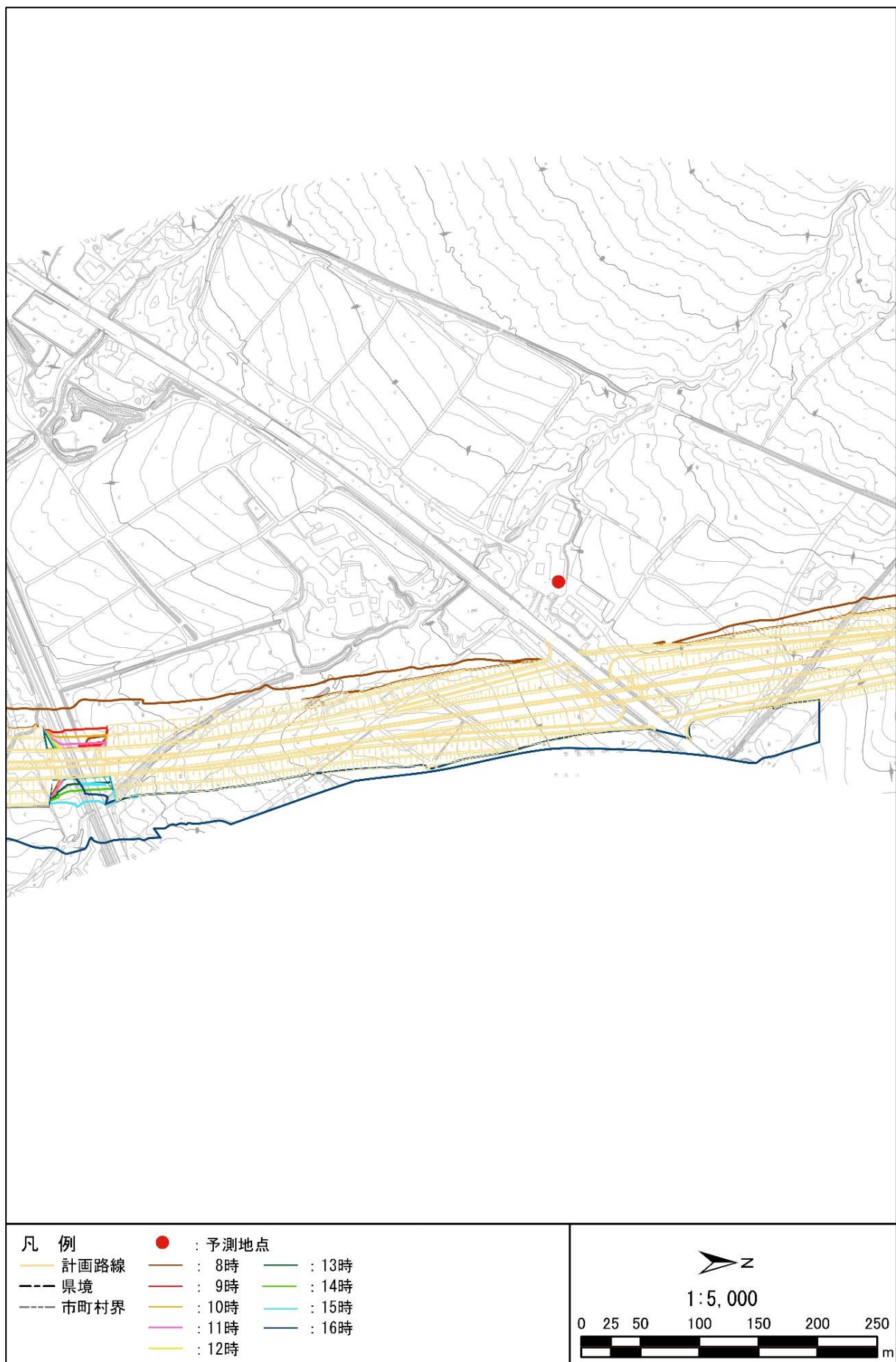
図 6.1-2(1) 等時刻日影図 (N1. 南牧村野辺山) (長野県)
