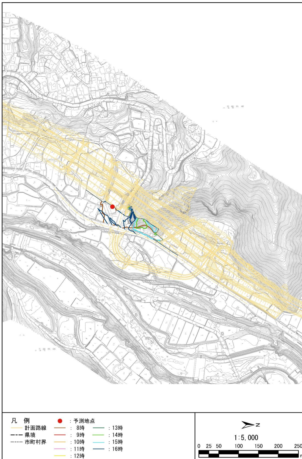
図 6.1-2 (3) 等時刻日影図 (N3. 小海町豊里 1) (長野県)
