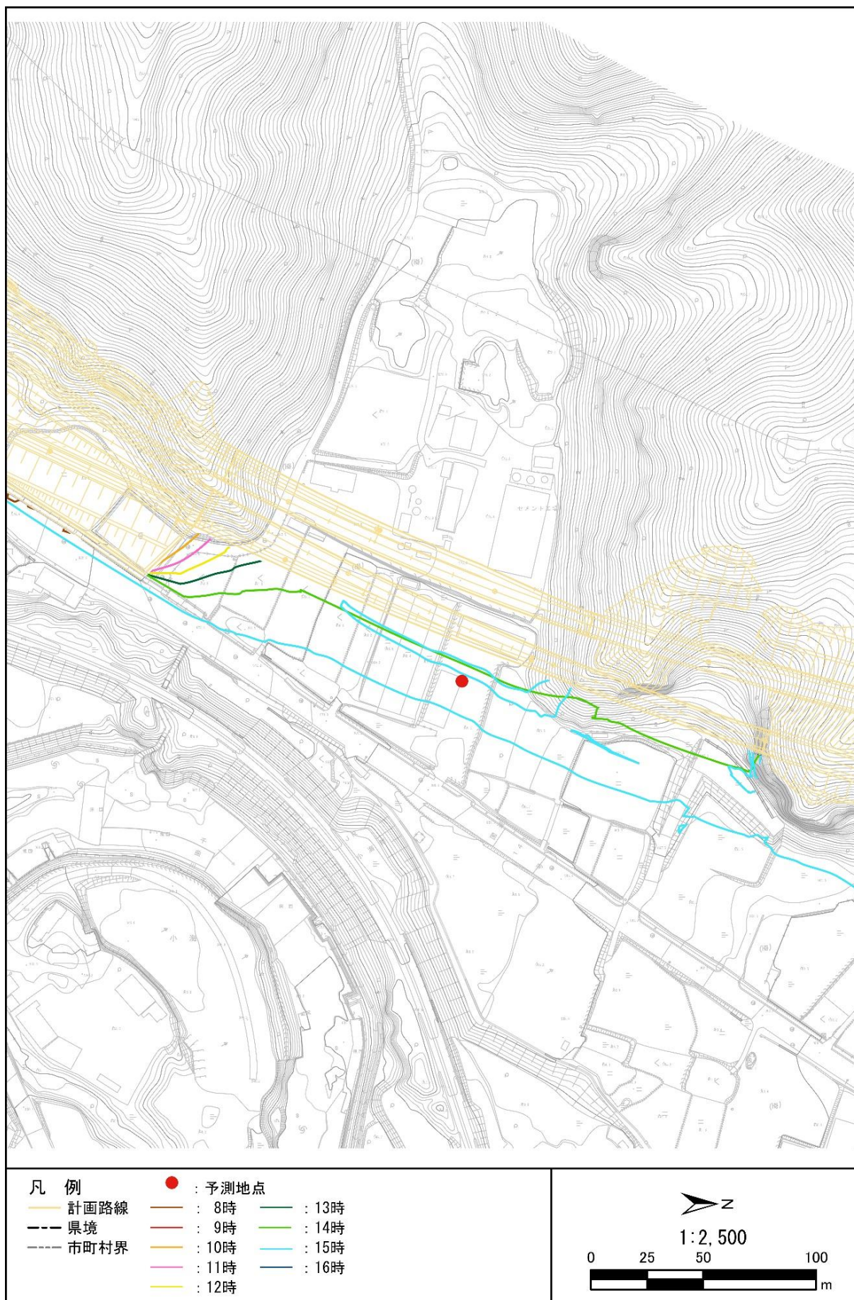
図 6.1-2(4) 等時刻日影図 (N4. 小海町豊里 2) (長野県)
