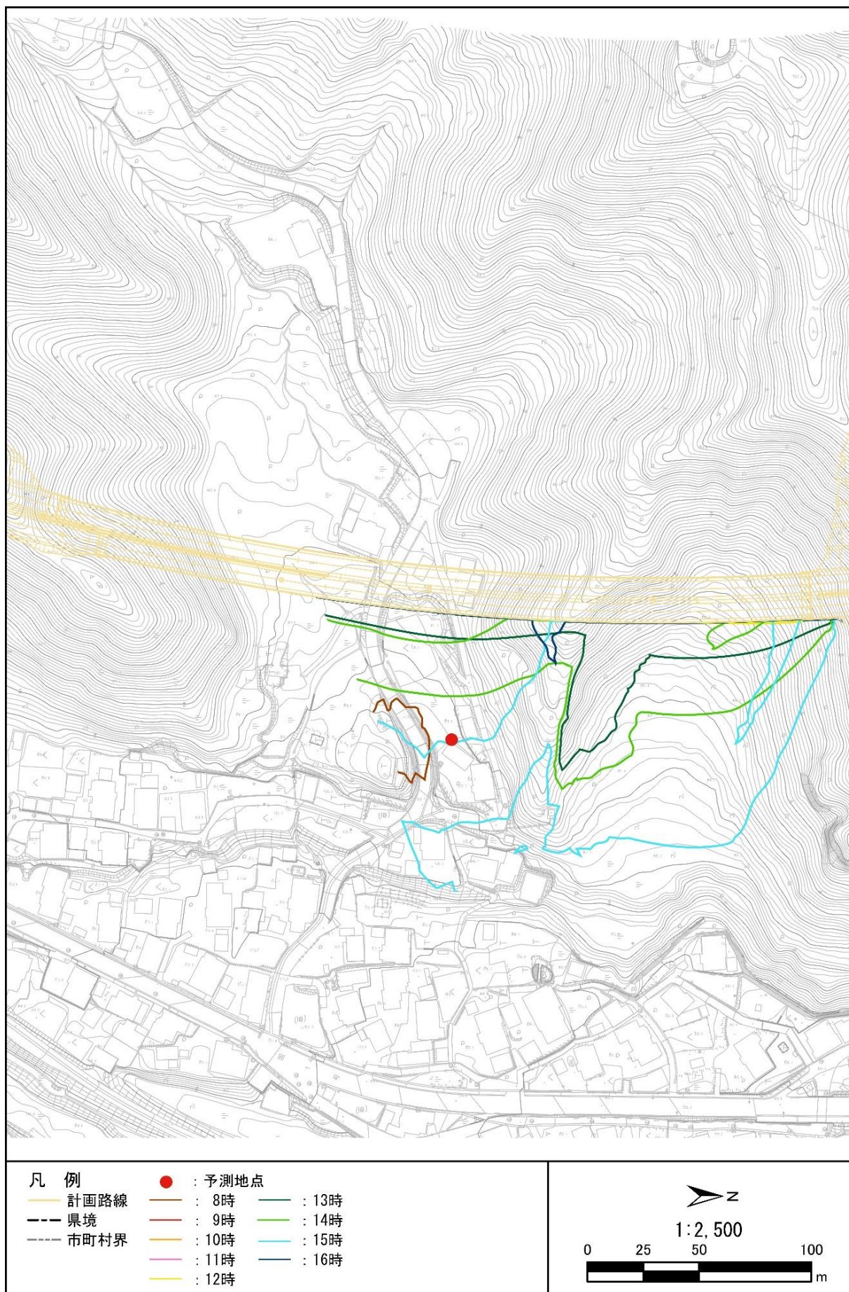
図 6.1-2(5) 等時刻日影図 (N5. 小海町豊里 3) (長野県)
