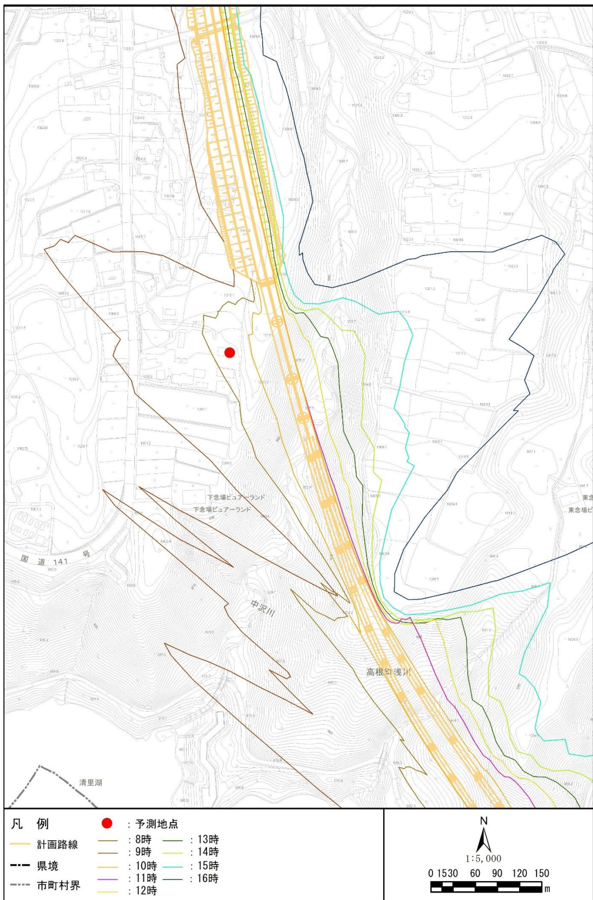
図 6.1-1(4) 等時刻日影図 (Y4. 高根町清里下念場) (山梨県)
