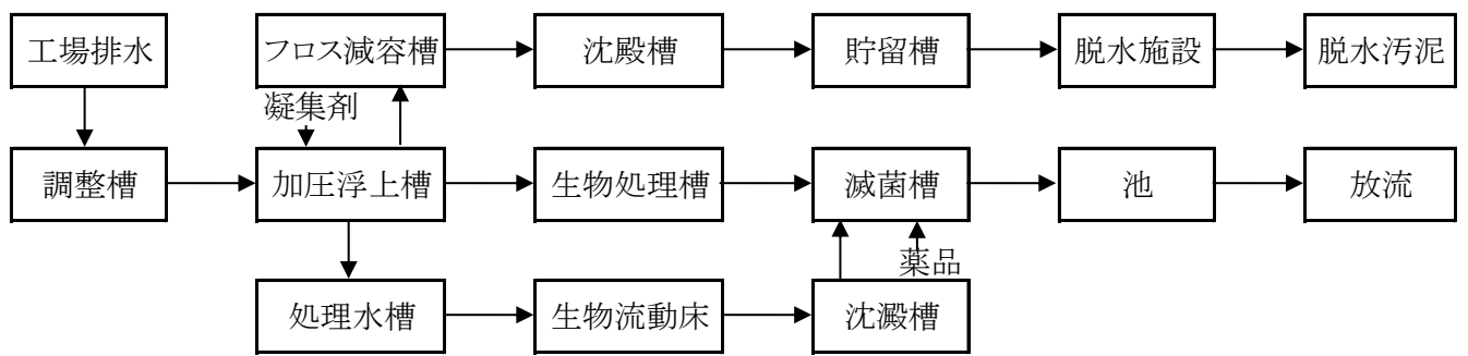
図 5 排水処理フローシート
