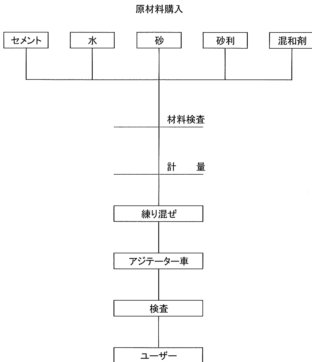
図1 製造工程
