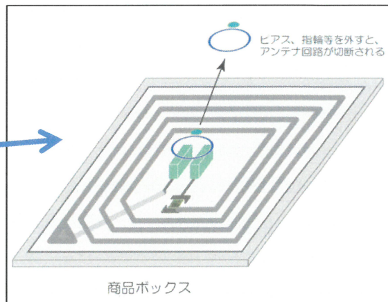
タグのスイッチ機構
