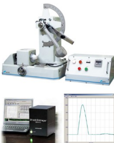
振子式衝撃試験機・加速度計測解析システム
