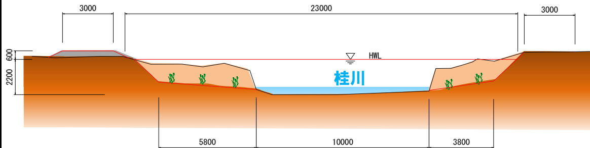
標準横断面図(イメージ)
