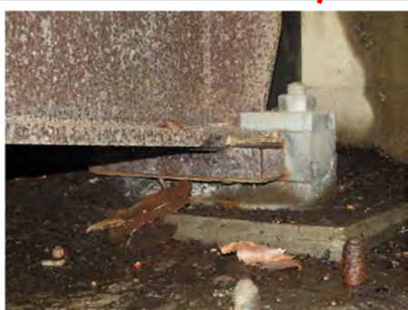
写真 1-6 支承 (腐食・土砂堆積)
