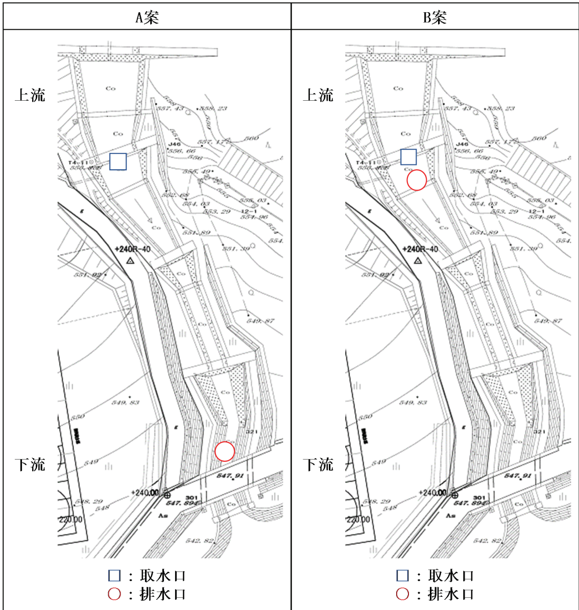
図3 取水口及び排水口の位置図 (A案及びB案)
