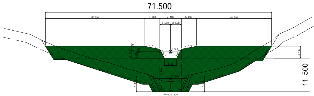
砂防堰堤 正面図
