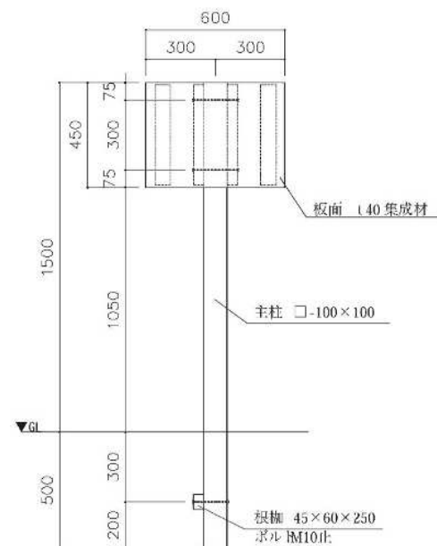
立面図
