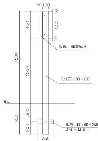
側面図
