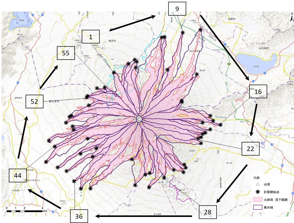
図 5.5-1 融雪型火山泥流のドリルマップ 計算開始点の配置一覧図
