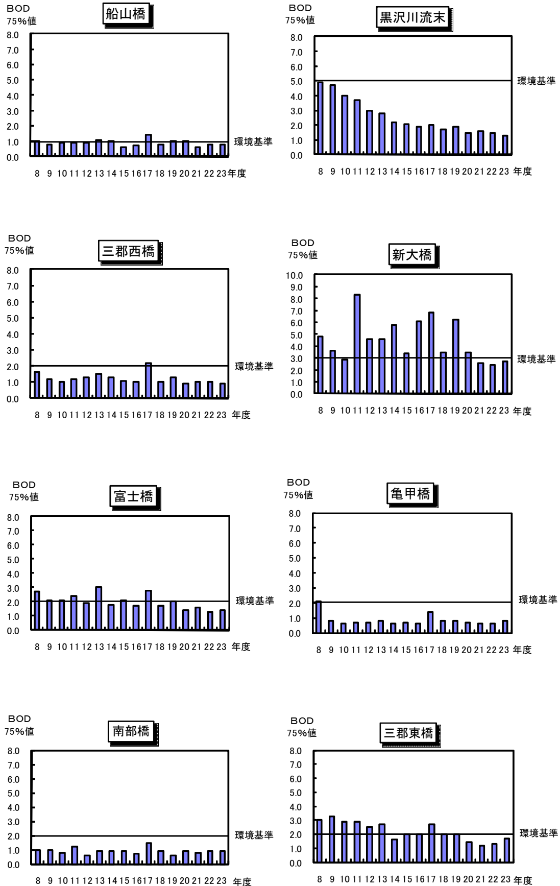
図－2 BOD（COD）75%値の推移
