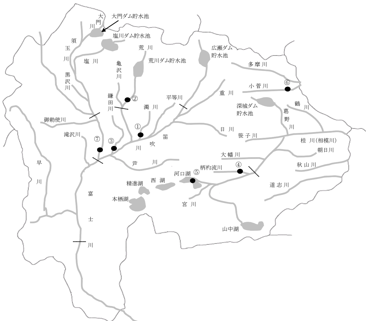
平成23年度ダイオキシン類常時監視地点図 公共用水域(水質・底質)
