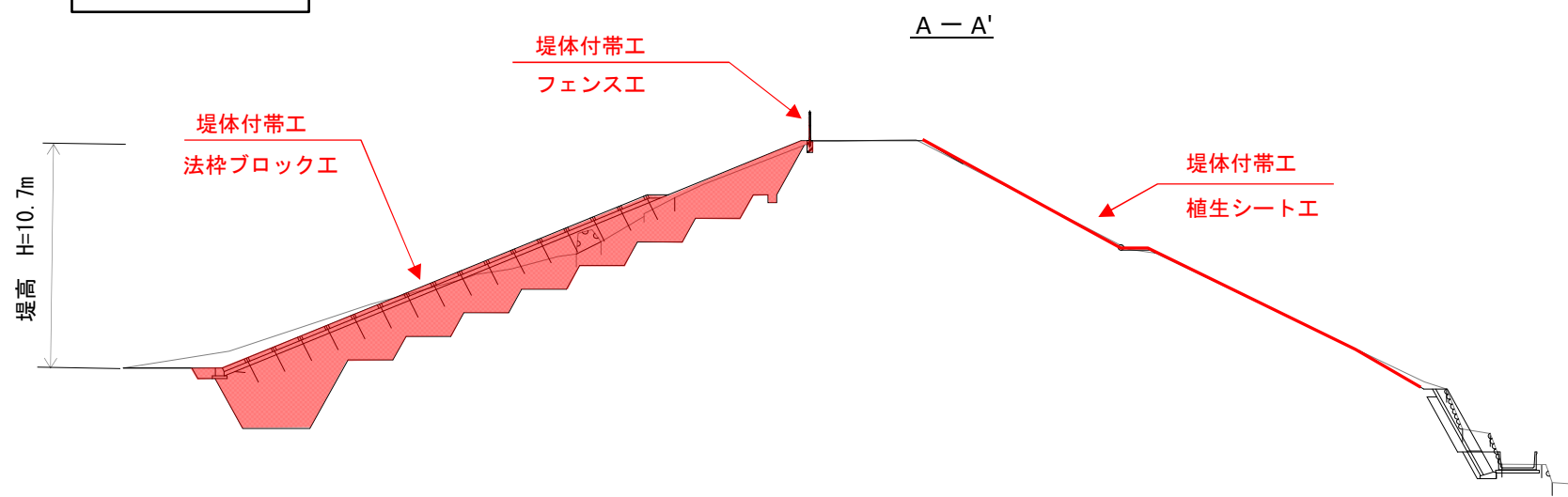
標準断面図
