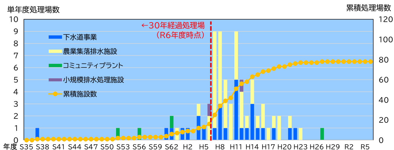
図 2 - 1 0 竣工年度度別の生活排水処理施設数（集合処理）
