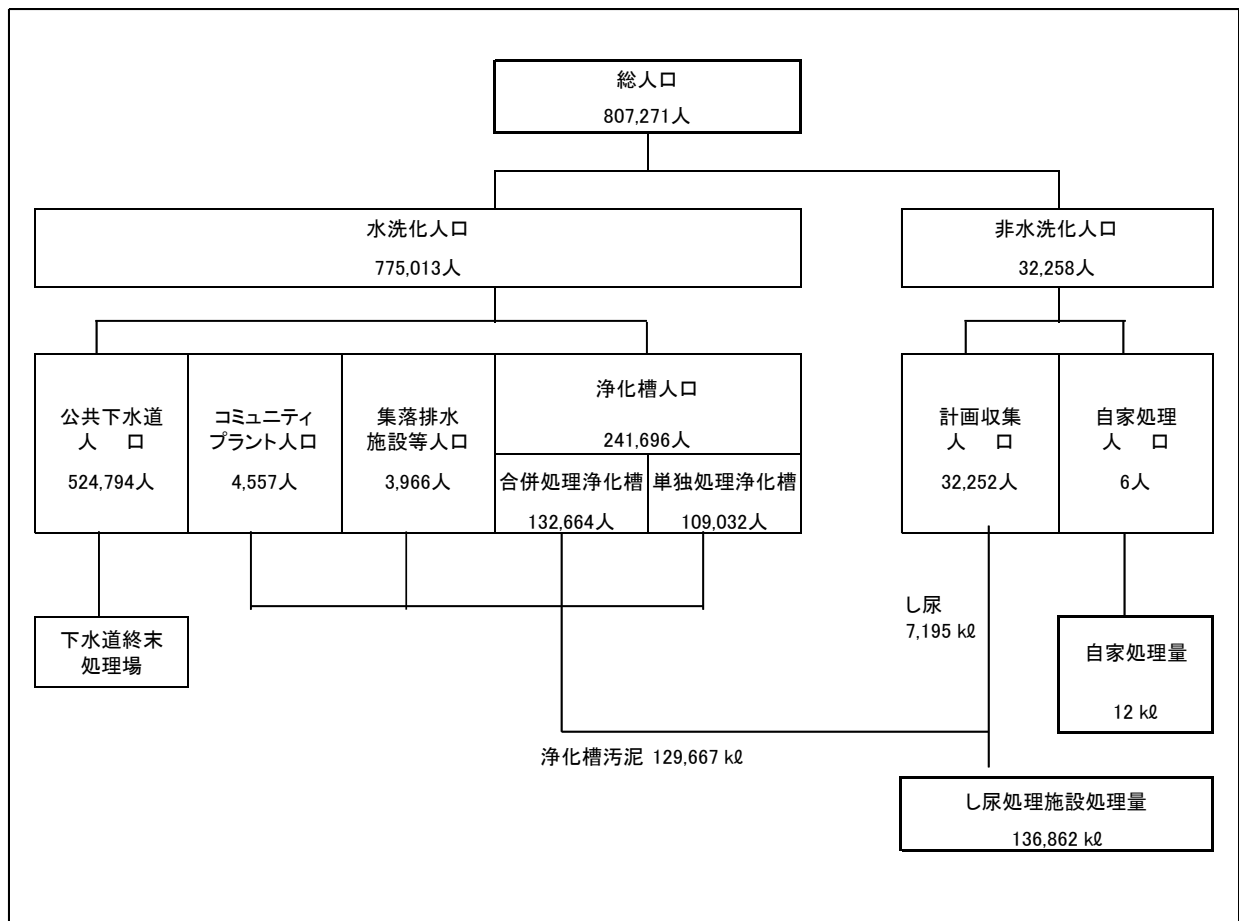
3-1 令和5年度し尿処理のフローシート
