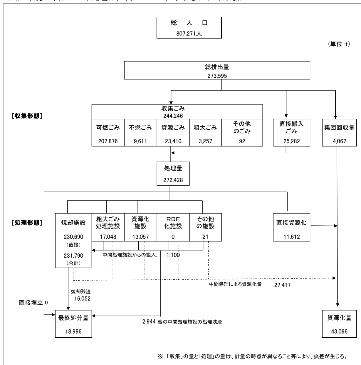
2-1 令和5年度ごみ処理のフローシート
