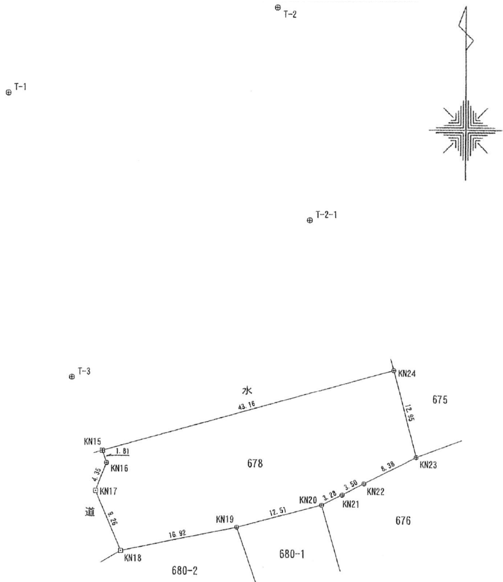
座 標 求 積 表
