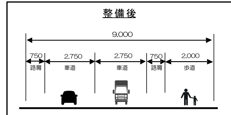
標準断面
