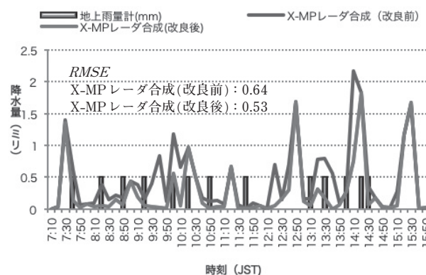
図2-8 富士山1合目におけるX-MPレーダ合成の改善前と改善後の推定値と地上雨量計実測値の時系列変化 (上図) 事例No.2 2013年7月23日 12:00～17:00JST (下図) 事例No.3 2013年7月29日 06:00～16:00JST
