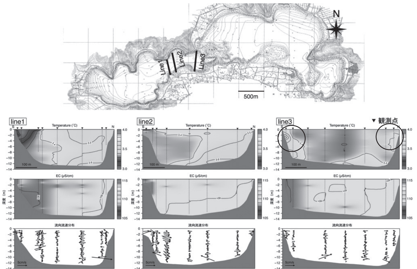
図4-3 河口湖における水質 (水温・電気伝導率)・流動状況の観測結果
