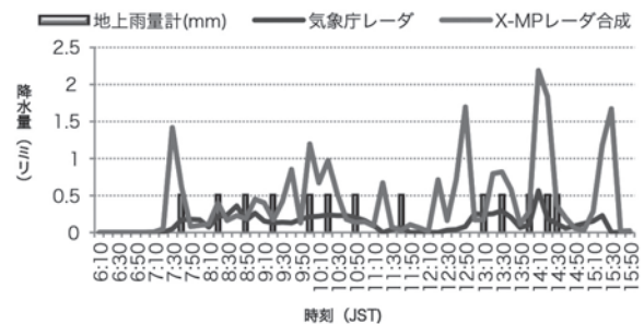
図2-5 富士山1合目におけるX-MPレーダ合成及び気象庁レーダの推定値と地上雨量計実測値の時系列変化 (上図) 事例No.2 2013年7月23日12:00~17:00JST (下図) 事例No.3 2013年7月29日06:00~16:00JST
