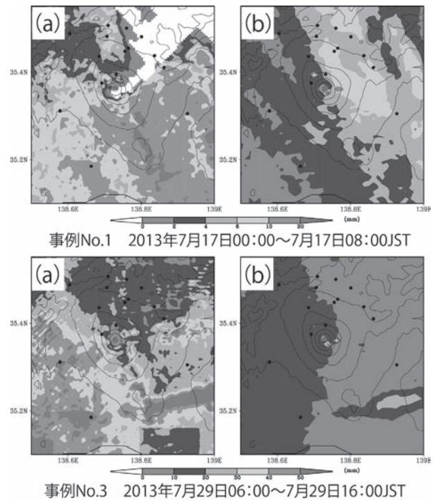
図2-4 各事例におけるX-MPレーダ合成と気象庁レーダの推定に基づいた積算降雨量分布図② (a) X-MPレーダ合成, (b) 気象庁レーダ
