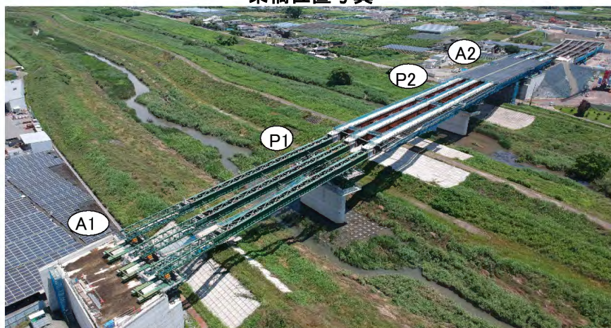
架橋位置写真
