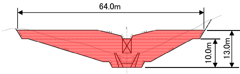
堰堤正面図
