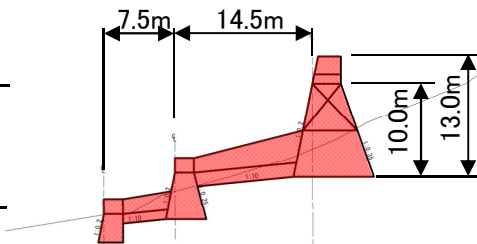
堰堤側面図
