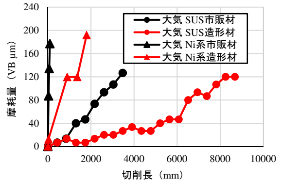
図2 切削加工性評価結果
