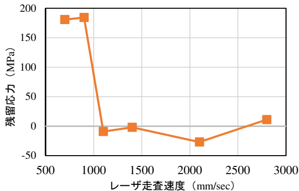
図1 残留応力測定結果
