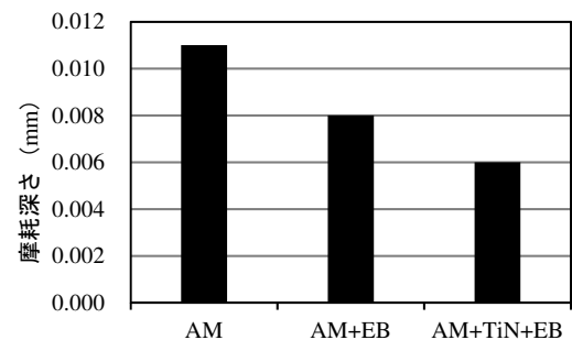
図3 摩擦摩耗試験結果
