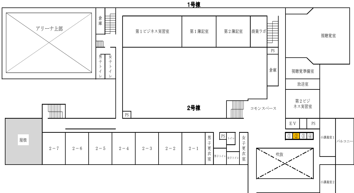
山梨県立富士北稜高等学校 1号棟・2号棟 3階平面図
