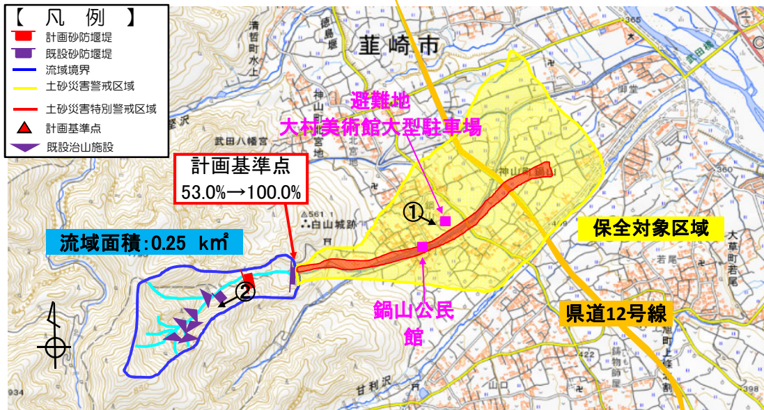
【流域概要図】
