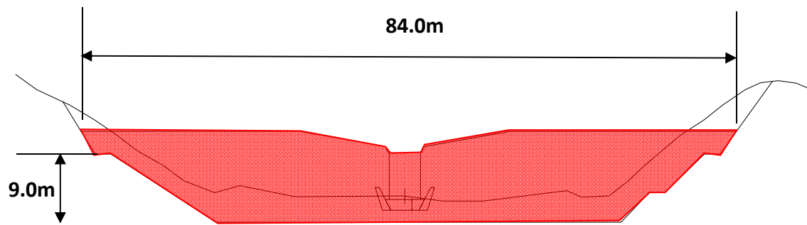
【堰堤正面図】
