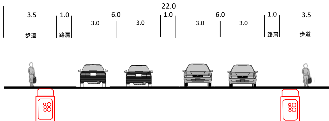
【標準横断図】
