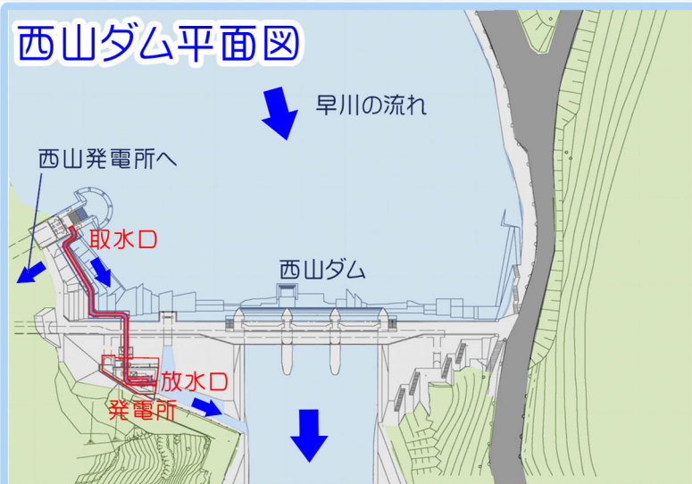
発電所平面図
