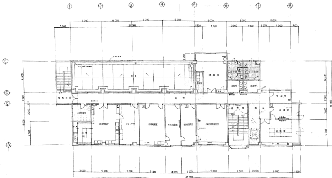
4階平面図
