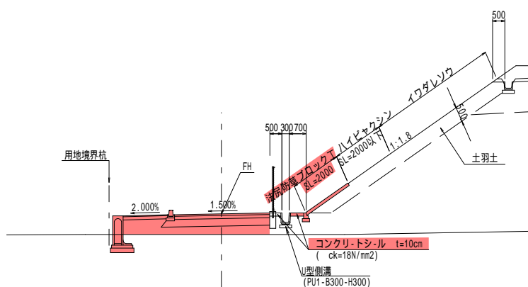
施工横断面図（側道）
