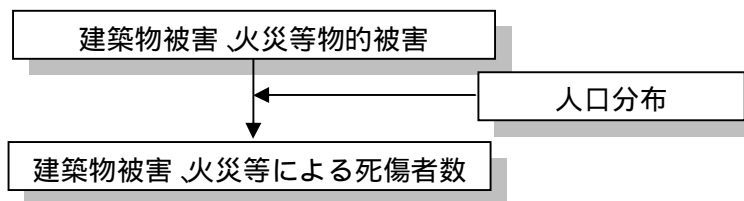
図 1-1 想定フロー
