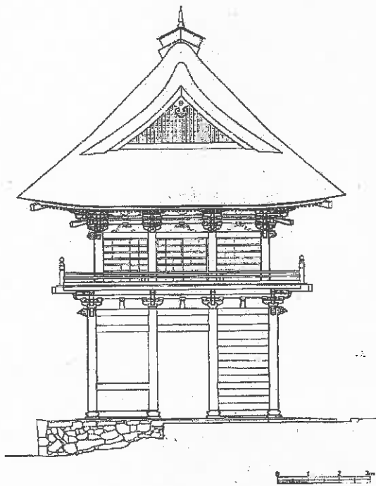
側面（東側）立面図
