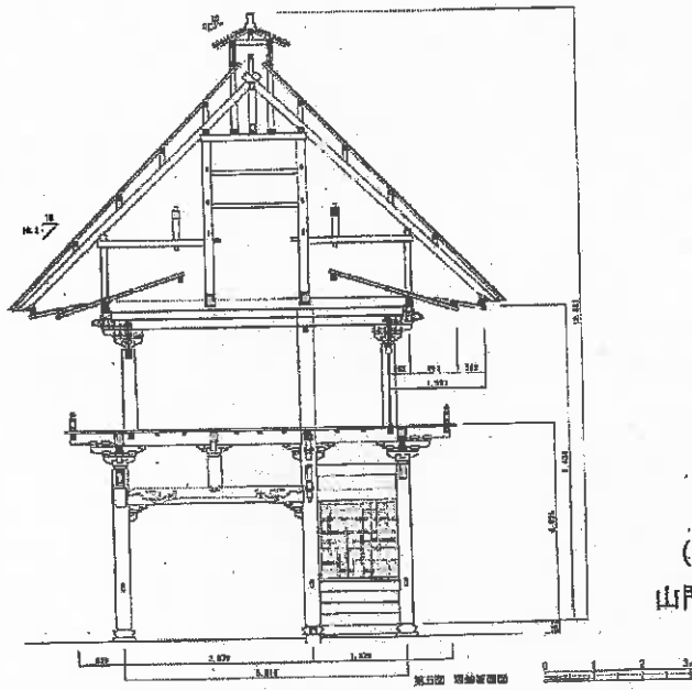
側面断面図
