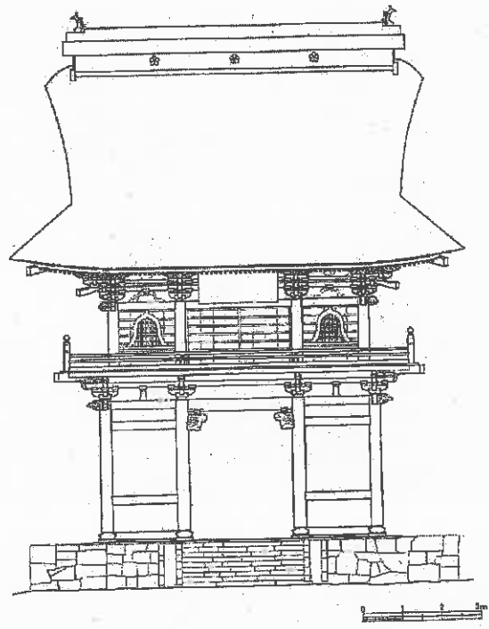
正面（南側）立面図
