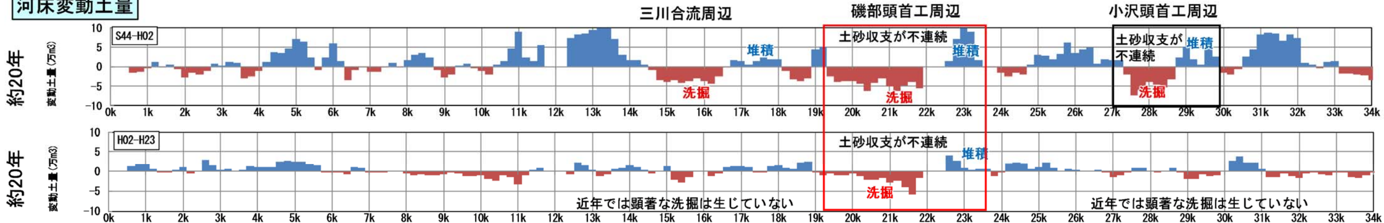
図 2.2.8 相模川 河床変動土量縦断面図
