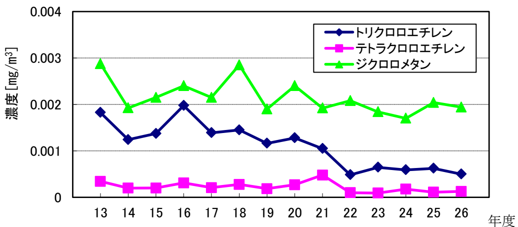
図10 トリクロロエチレン、テトラクロロエチレン及びジクロロメタンの年平均値の経年変化
