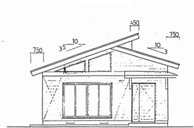
北側立面图
