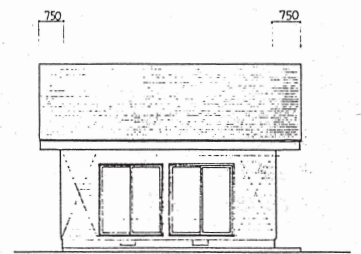
東側立面图
