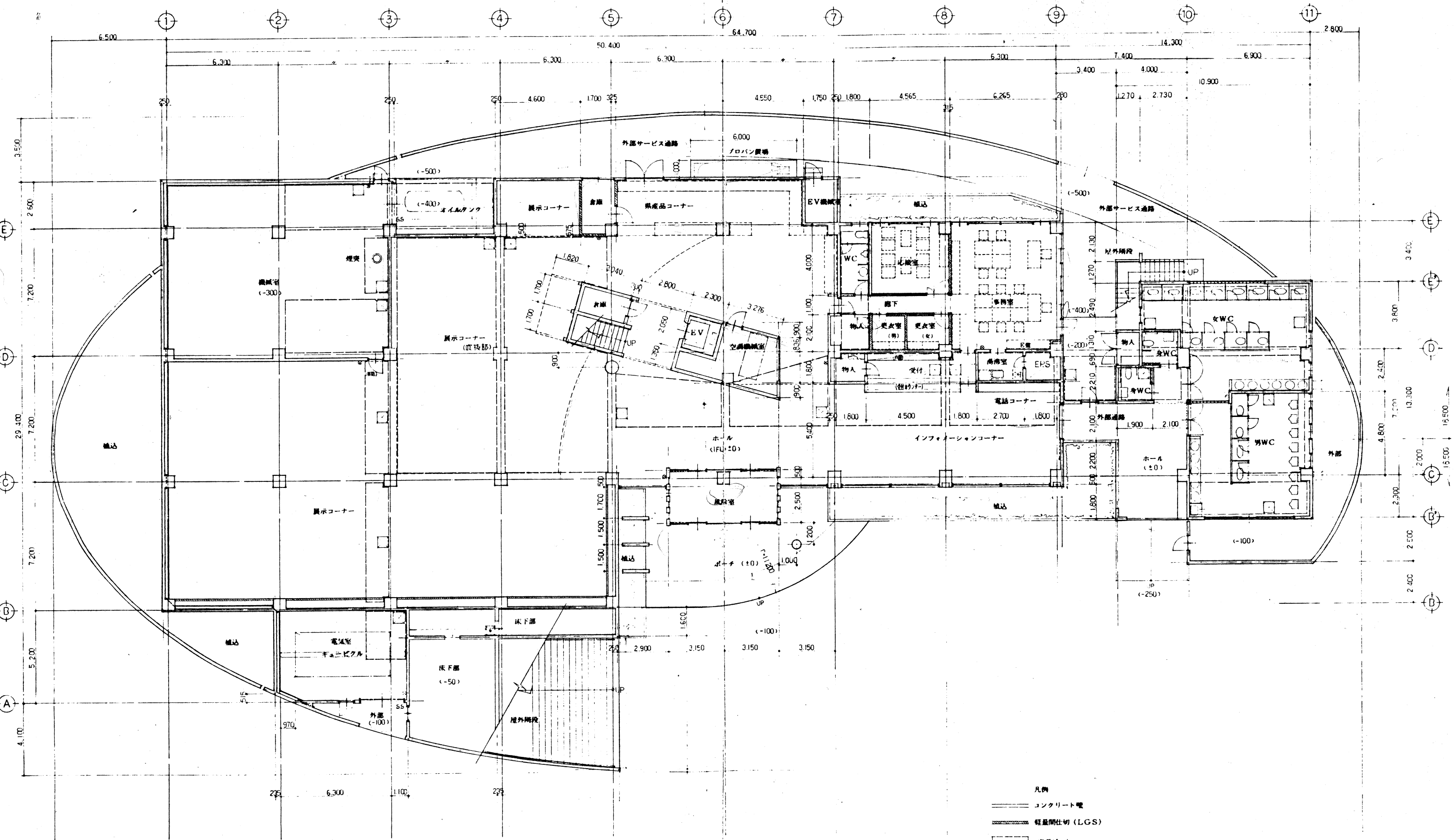
1階 平面図 5.1/100
